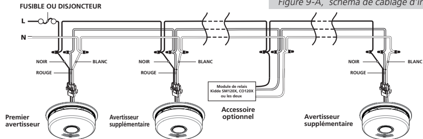
Figure 9-A, schéma de câblage d'interconnexion
